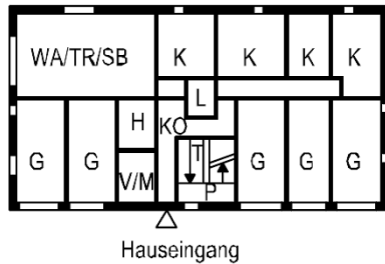
Vollgeschoss / Erdgeschoss
